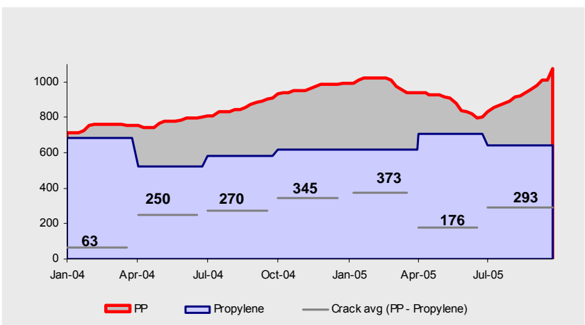
Polypropylene ; EUR/ton
