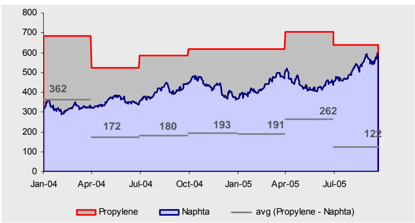
Polypropylene ; EUR/ton
