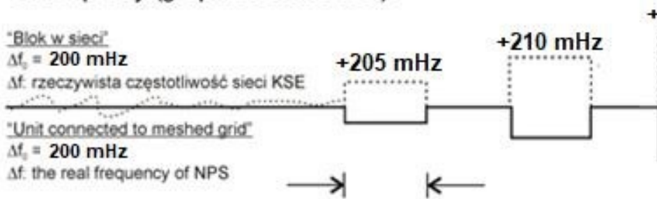
Rys. 1 Sprawdzenie niewrażliwości odpowiedzi częstotliwościowej.
