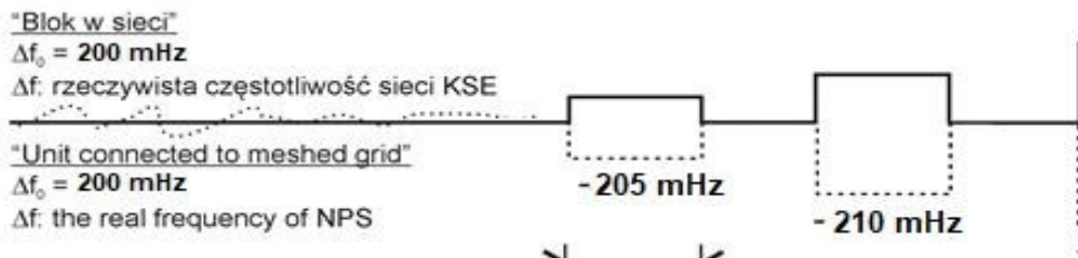
Rys. 1 Sprawdzenie niewrażliwości odpowiedzi częstotliwościowej.
