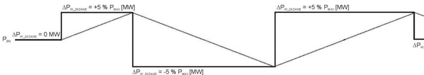
Rys. 4 sprawdzenie działania regulacji wtórnej w odpowiedzi na wymuszenie w torze regulacji wtórnej w trakcie wyłączania i załączania stanu regulacji wtórnej
